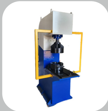
Hydraulic C Press
